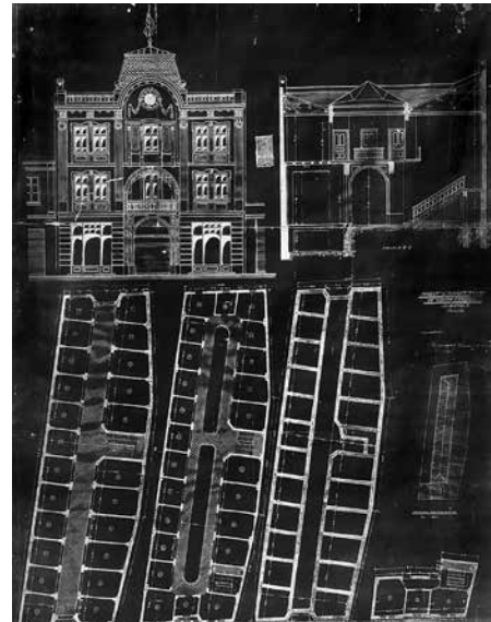
Безистенът в Бургас, проектиран 25.02.1922 г. Вдясно: План за Безистена от арх. Славоф & Тоскани
